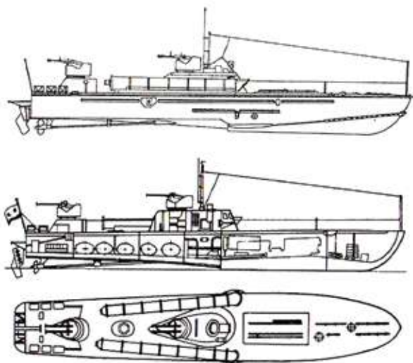
Чертежная схема «Комсомольца»
